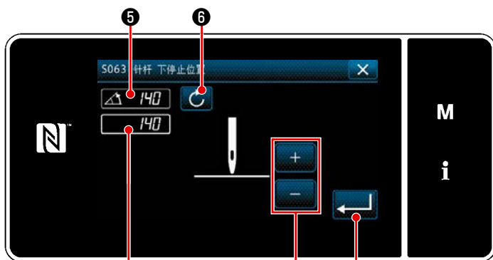
< 针杆下停止位置设定画面 >
