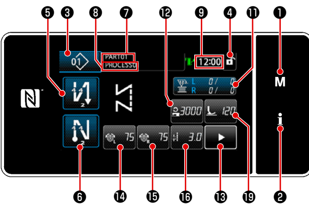
自由缝纫图案（操作人员模式）
