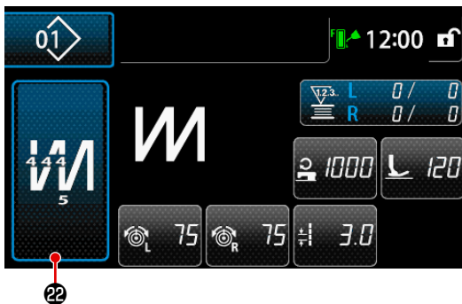
重叠缝纫图案（操作人员模式）
