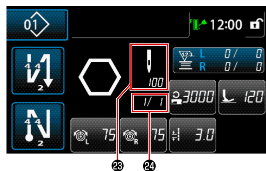
多角缝纫图案（操作人员模式）
