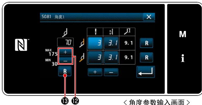
＜角度参数输入画面＞
