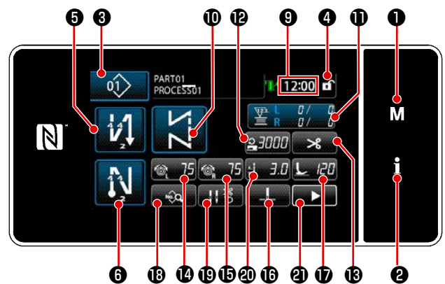
固定尺寸缝纫图案（操作人员模式）
